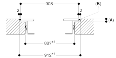
Coupe longitudinale
