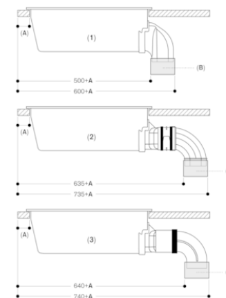
1: Installation directe 2: Installation avec rallonge pour plan de travail très profond et conduit plastique : - AD 851 041 (pièce de connexion pour rallonge) - AD 857 040 (pièce de connexion à gaine plate, plastique) - AD 857 030 (coude de gaine plate, 90°, vertical, plastique) 3: Installation avec rallonge pour plan de travail très profond et conduit en métal : - AD 851 041 (pièce de connexion pour rallonge) - AD 854 000 (pièce de connexion à gaine plate, métal) - AD 854 030 (coude de gaine plate, 90°, vertical, métal)
