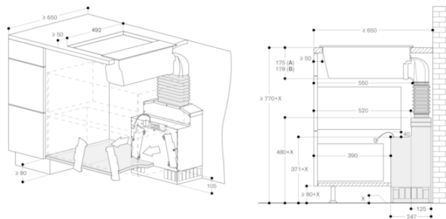
A: Montage sur le plan de travail B: Montage à fleur de plan (VL414 uniquement) Mesures en mm
