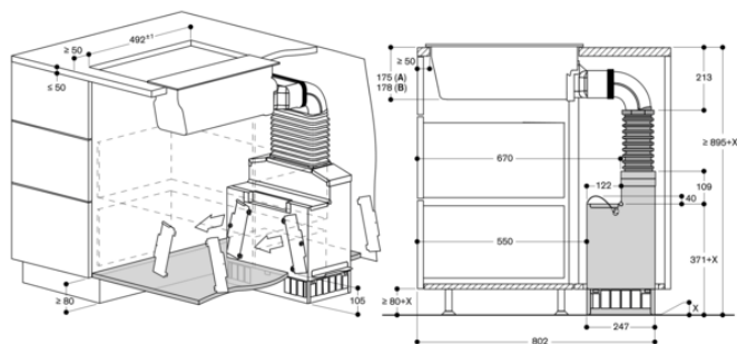
A: Montage sur le plan de travail B: Montage à fleur de plan (VL414 uniquement) Mesures en mm
