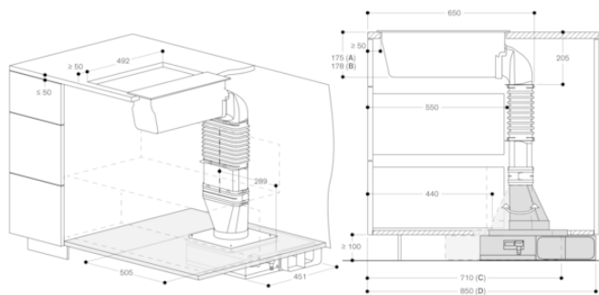
A: Montage sur le plan de travail B: Montage à fleur de plan (VL414 uniquement) C: Évacuation vers la gauche. Pièce de connexion plate/ronde placée vers l'avant D: Évacuation vers la droite. Pièce de connexion plate/ronde placée vers l'arrière Mesures en mm
