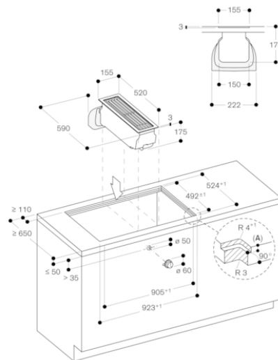
A: 3.5 -0.5 6.5 +0.5 en combinaison avec les plaques de cuisson à induction Mesures en mm
