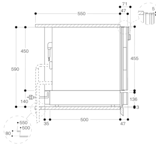
Vue de côté WS 461 sous BS, BM, CM
